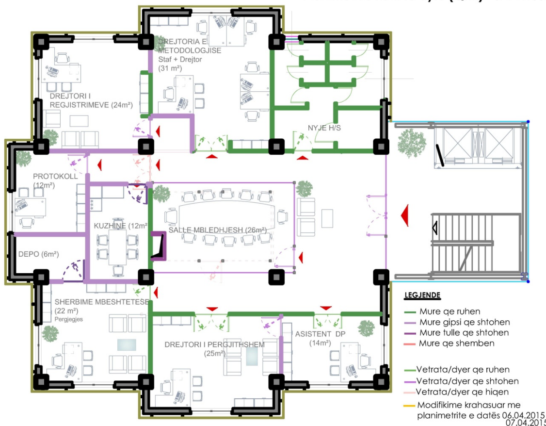
Planimetri e katit të dytë (QKR) - Sh. 1:100
